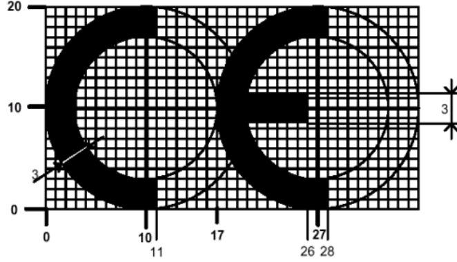
Şekil 7: "CE" İşaretinin Şekli
